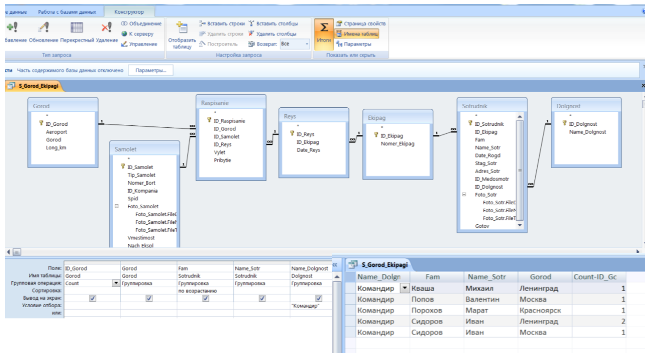
Рисунок 6 - Бланк запроса Goro_Ekipagi и результаты его выполнения
