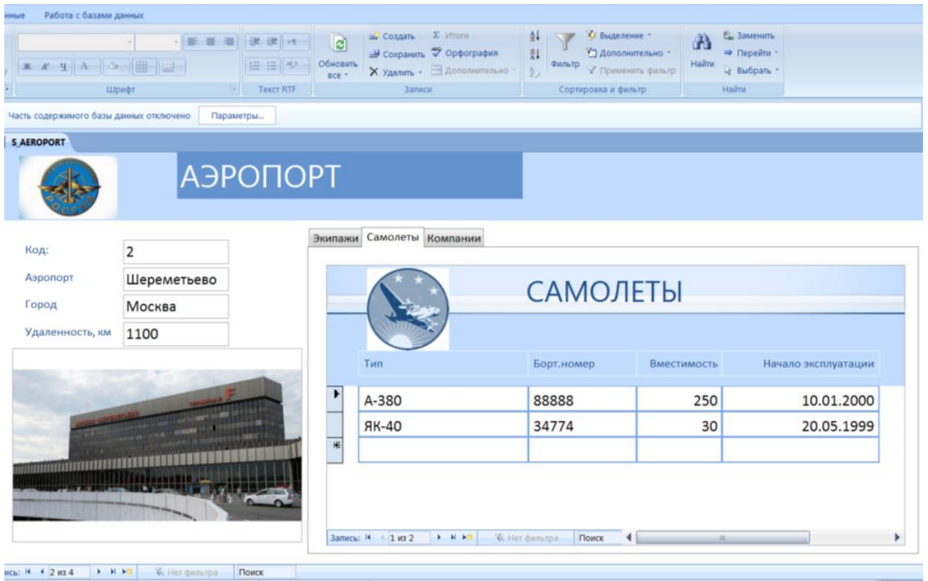
Рисунок 15 - Форма Аэропорты с открытой вкладкой Самолеты
